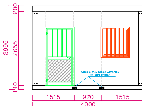
PROSPETTO 1
