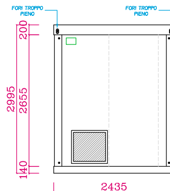
PROSPETTO 2
