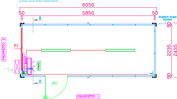
PIANTA GENERALE
