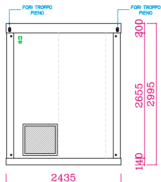
PROSPETTO 3
