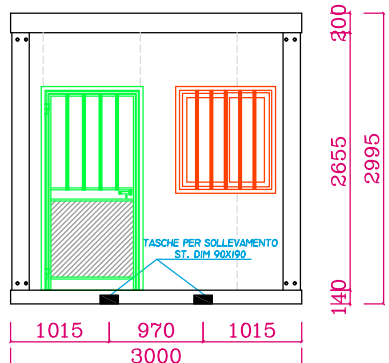
PROSPETTO 1
