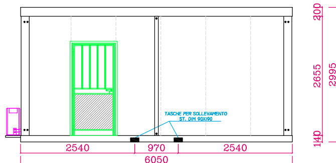
PROSPETTO 1
