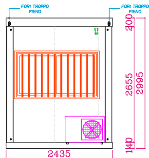
PROSPETTO 2
